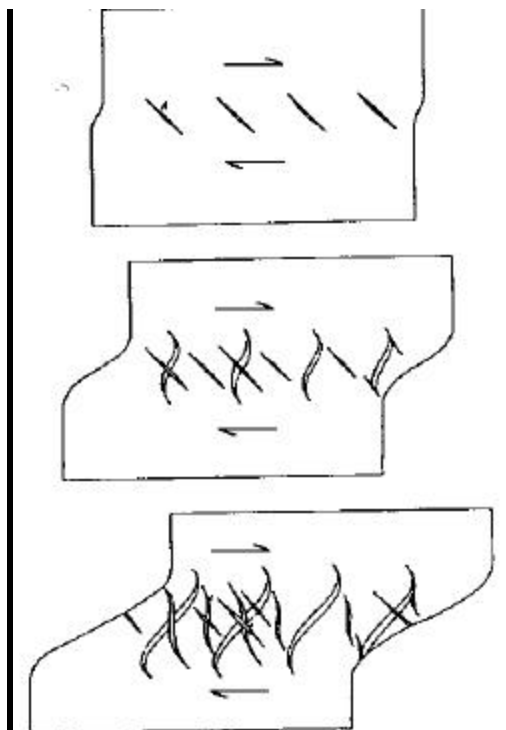
Figura 14. Las vetillas escalonadas y su relación con los bordes de la zona de cizalla. Nótese la formación de distintas generaciones durante la deformación progresiva (Durney y Ramsay 1973, Fig. 15)
